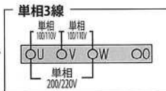
カムスイッチ (三相⇄単相切替)
