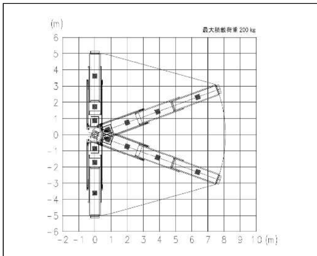
SF77A-IV 作業範囲図 プラットフォーム
