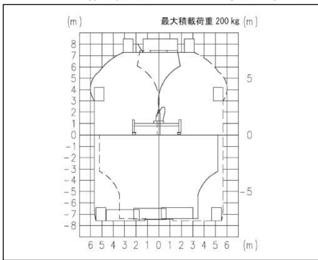
SF77A-IV 作業範囲図 アウトリガ張出量最大
