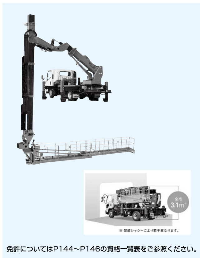
SF77A-IV 作業範囲図 アウトリガ張出量最大
